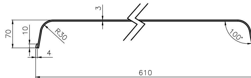
A-A断面图 (1/5)
