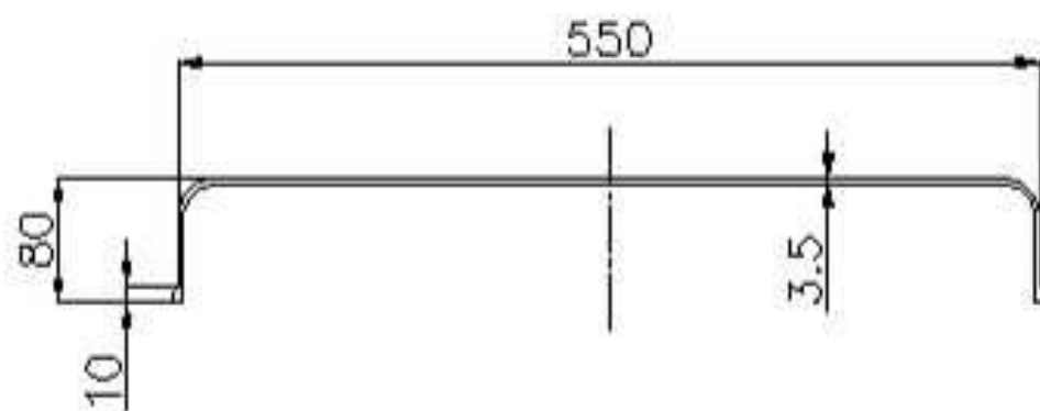
A-A断面图
