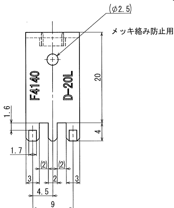
プリント基板加工例 t=1.6
