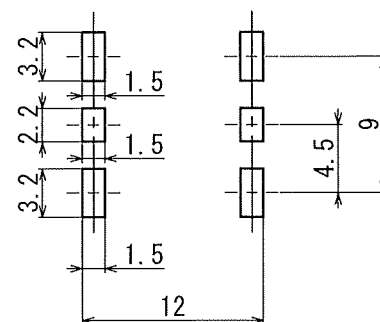
プリント基板加工例 t=1.6
