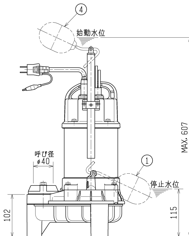
No. 1 ポンプ
