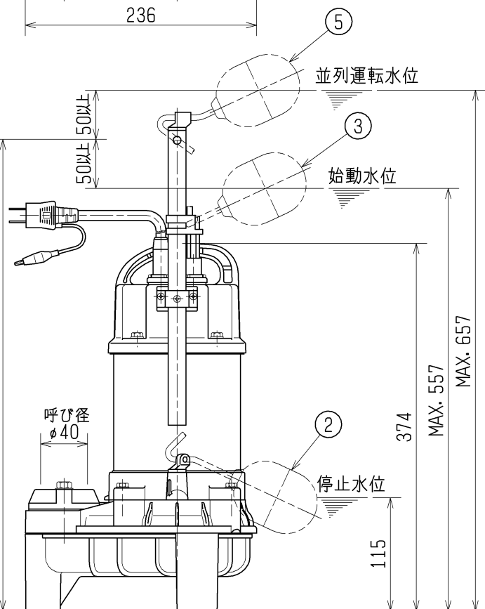
No. 2 ポンプ
