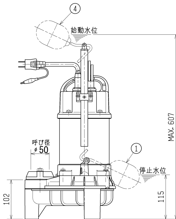
No. 1 ポンプ
