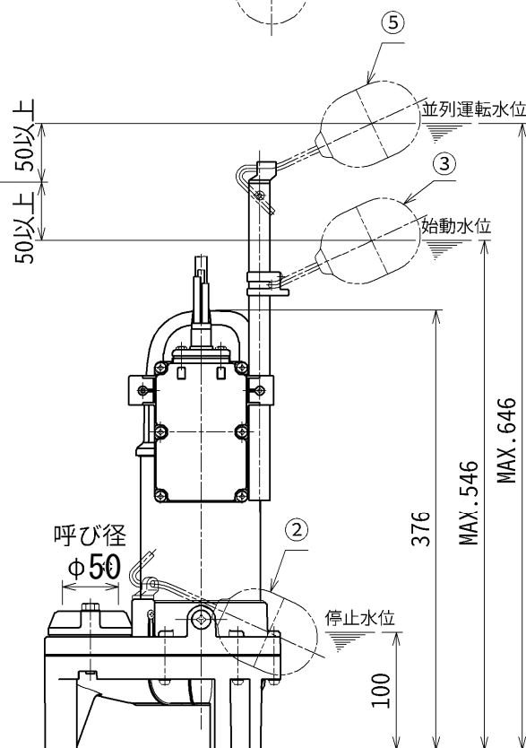
No.2 ポンプ
