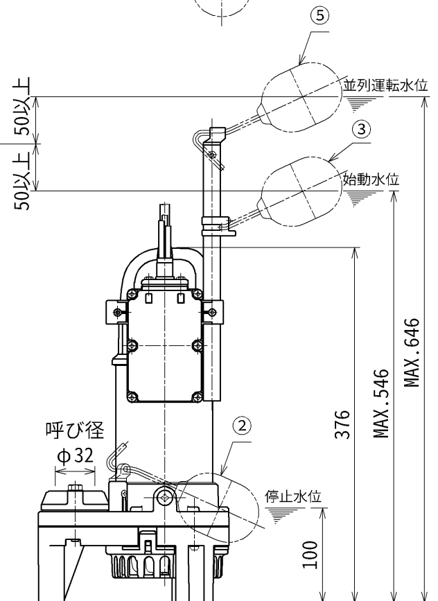
No.2 ポンプ
