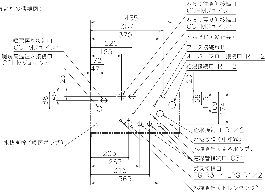
■A部詳細図(尺度1/5)
