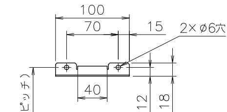
■A部詳細図(尺度1/5)
