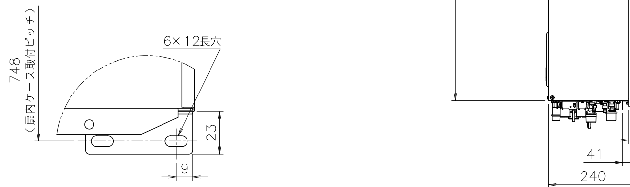
■B部詳細図 (尺度 1/2)
