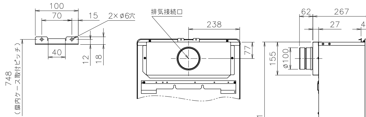
■B部詳細図(尺度1/2)
