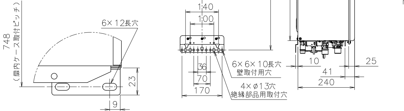
■B部詳細図(尺度1/2)
