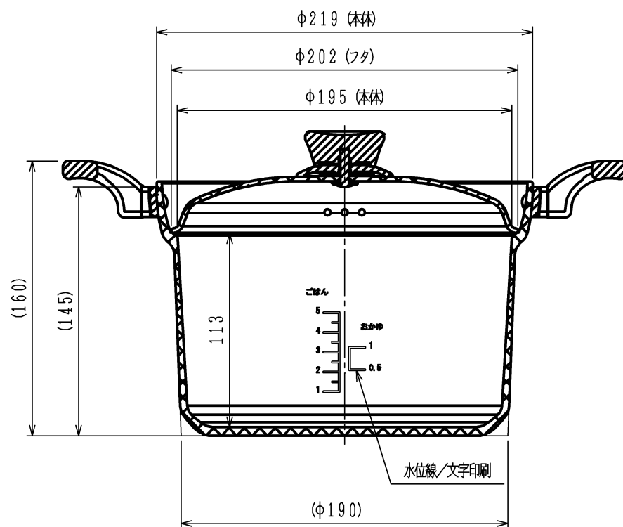
AA断面図
