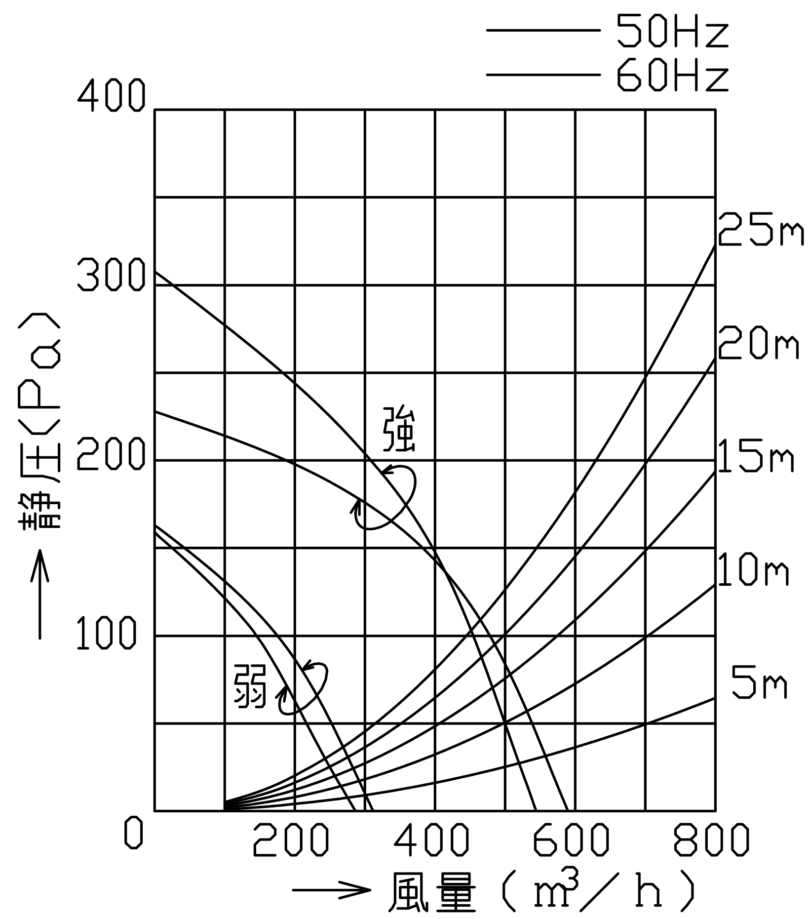
静圧－風量 曲線
