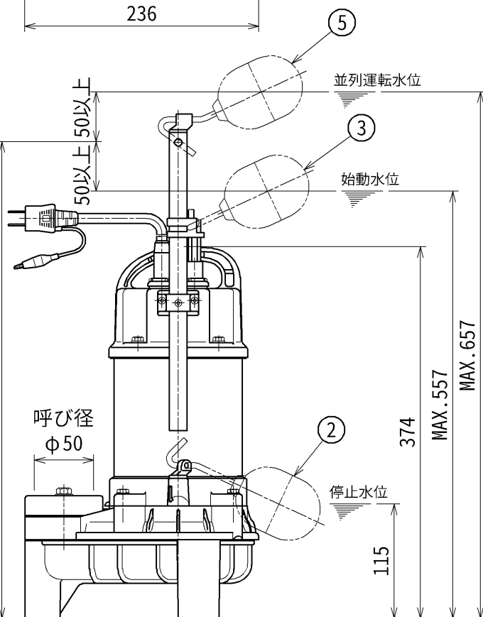
No.2 ポンプ
