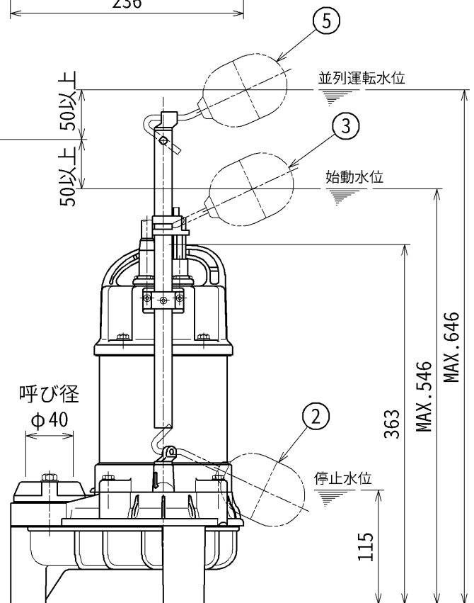
No.2 ポンプ
