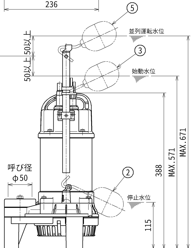
No.2 ポンプ
