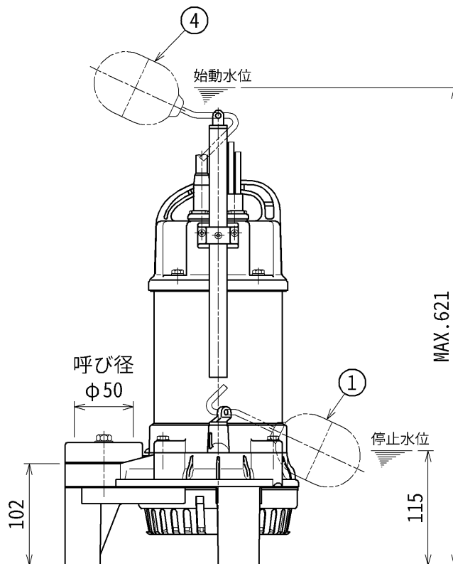
No.1 ポンプ
