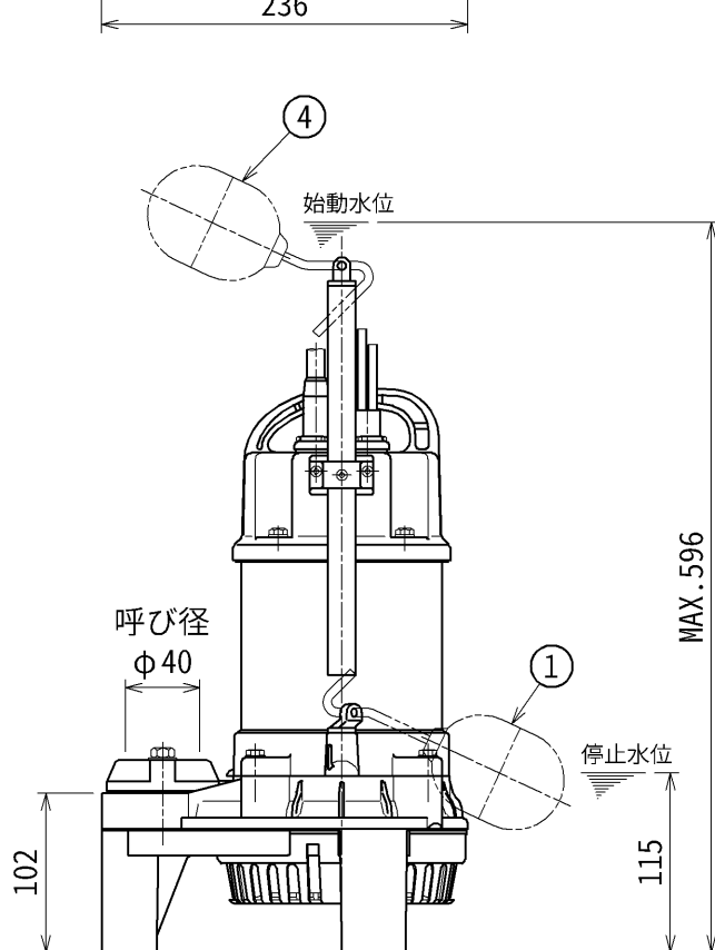
No.1 ポンプ
