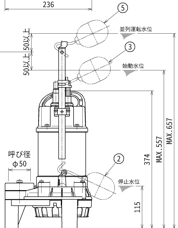
No.2 ポンプ
