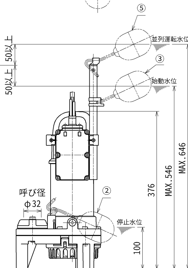
No.2 ポンプ
