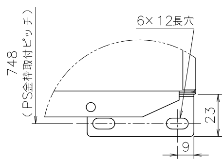
■B部詳細図（尺度1／2）
