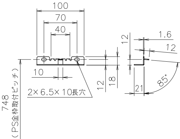
■B部詳細図（尺度1／2）
