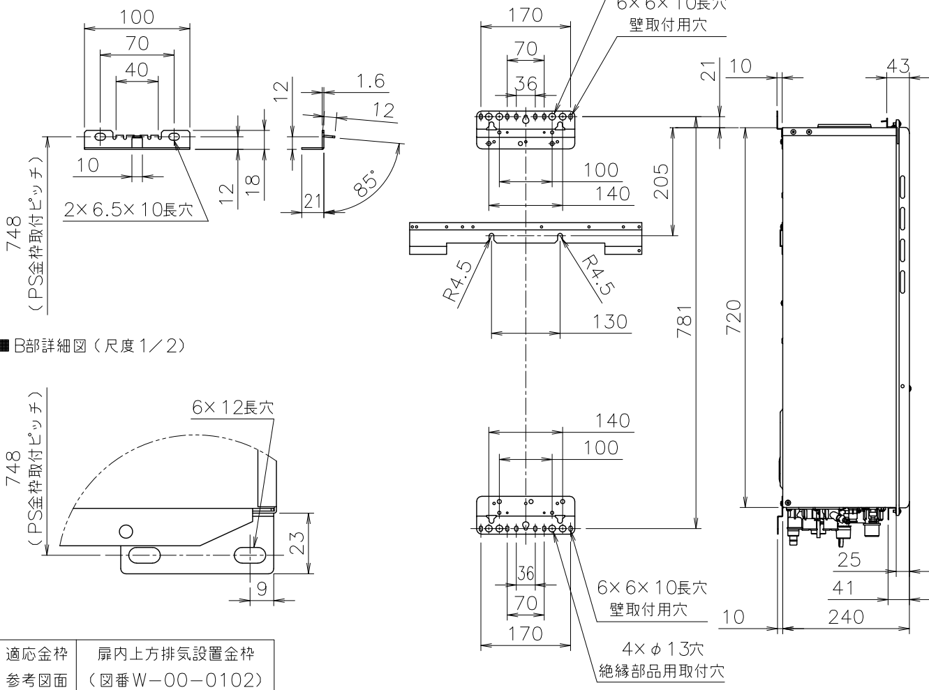
■A部詳細図(尺度1/5)
