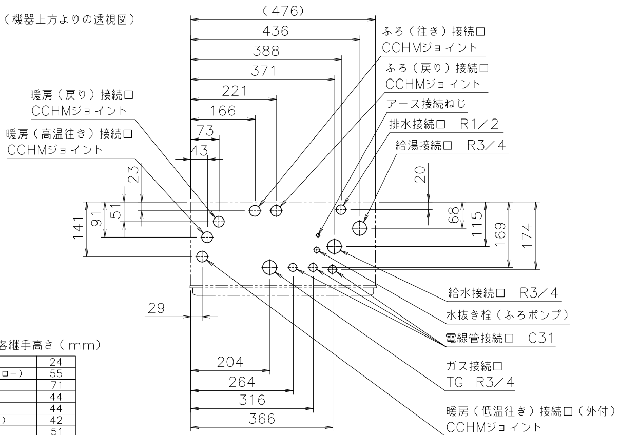
■A部詳細図（尺度1／5）
