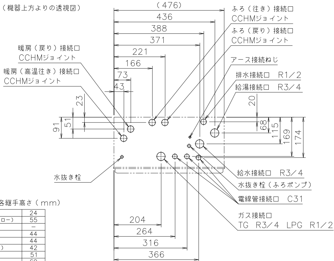
■A部詳細図（尺度1／5）
