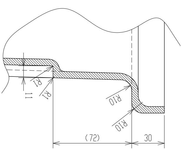
A部詳細図 (S=1:2)
