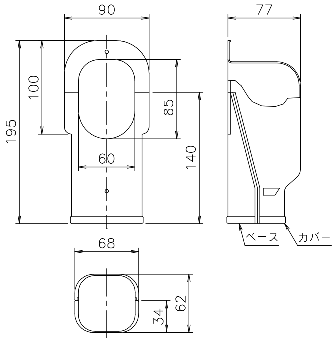
⑥ ウォールコーナー SW-66 材質：PVC 色：アイボリー （S=1/4）
