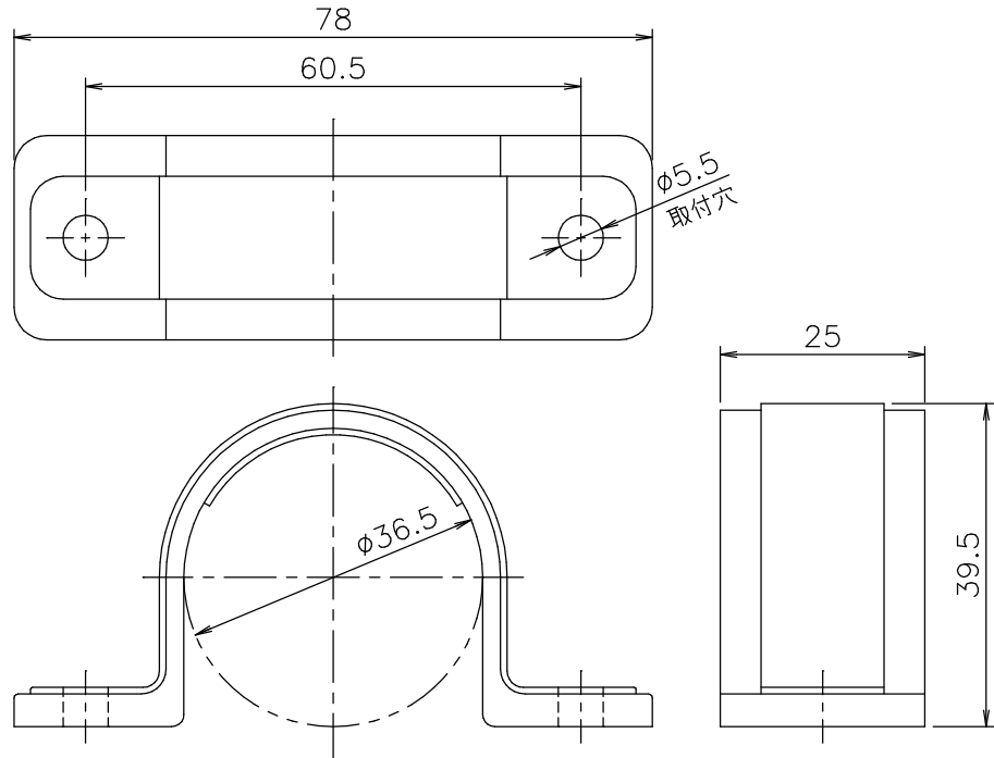
⑧ サドルバンド 30用 材質：PVC 色：アイボリー
