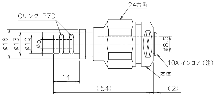
⑤ CHP1-10W（10Aインコア含む） 材質：黄銅（C3604BD）
