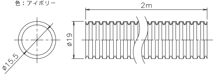
⑨ 遮熱管 2m 色：アイボリー
