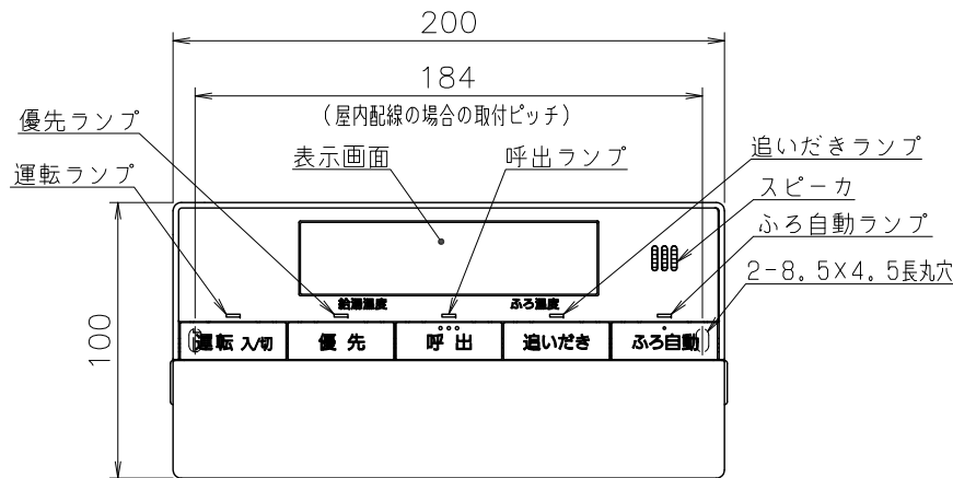
浴室リモコン RC-J101S
