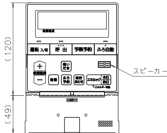
浴室リモコン RC-J101S
