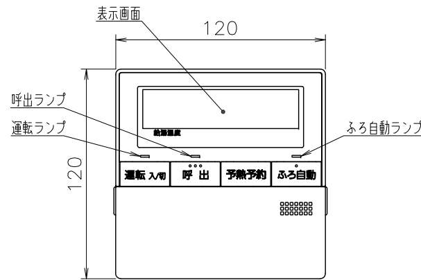
台所リモコン RC-J124M
