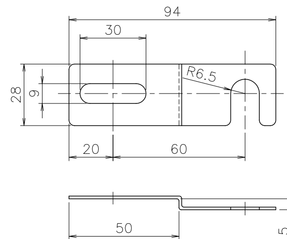
■ 本体固定金具（尺度1／3）
