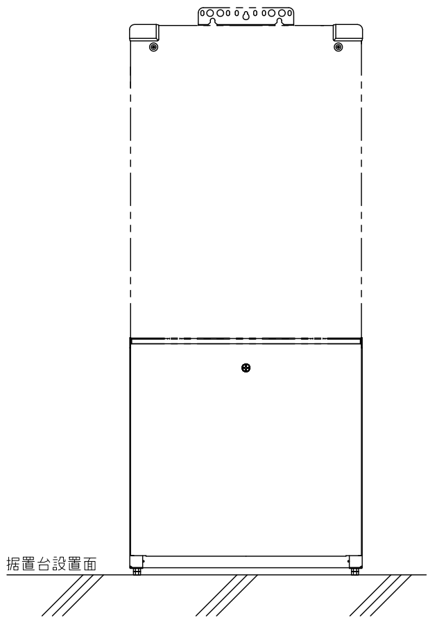
■設置例 (尺度 1/10)
