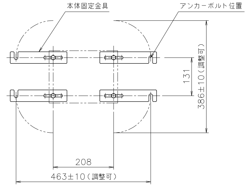
（上方よりの透視図）（尺度 1／10）
