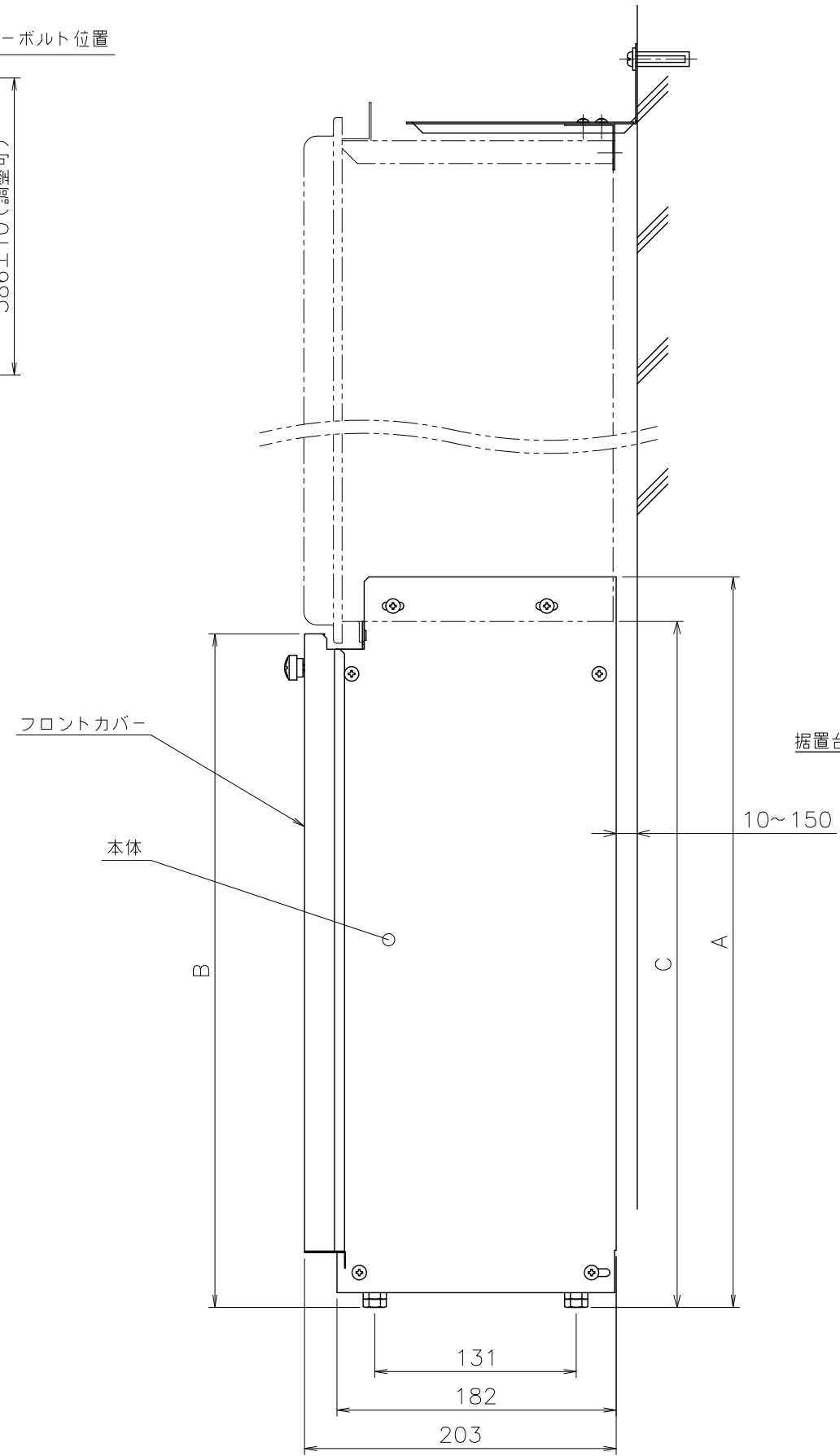
■設置例（1／10）
