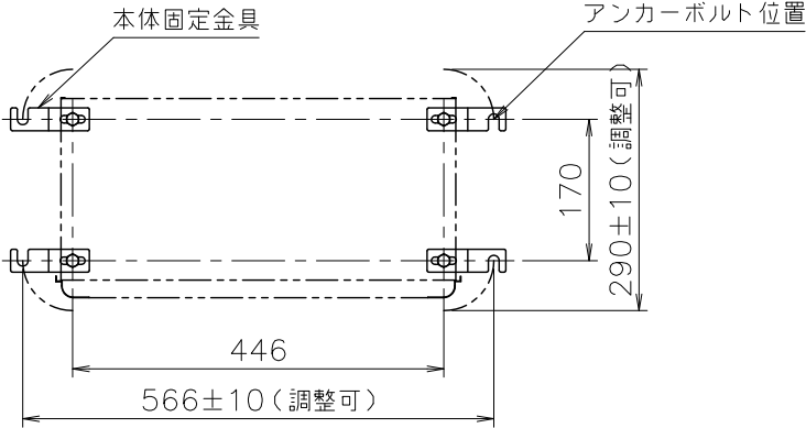
（上方よりの透視図）（尺度 1／10）
