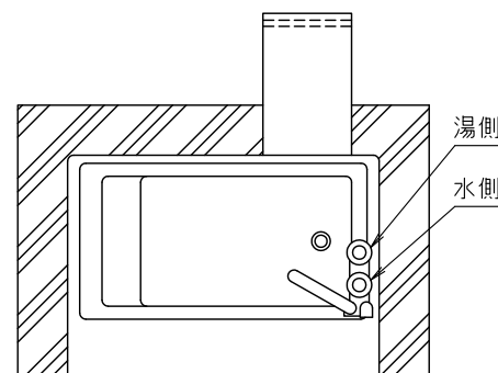
■浴槽取付例（Rタイプ）
