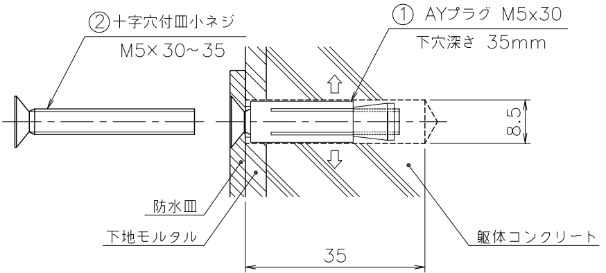
A部施工例（3箇所） スケール 1：1 （①及び②は現場手配）
