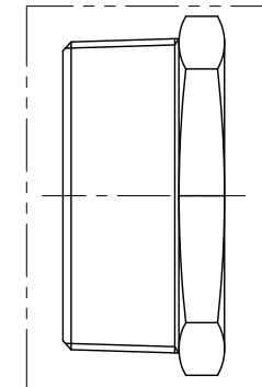
側面吸込金物 C2 25Aのみ付属 材質：SCS13
