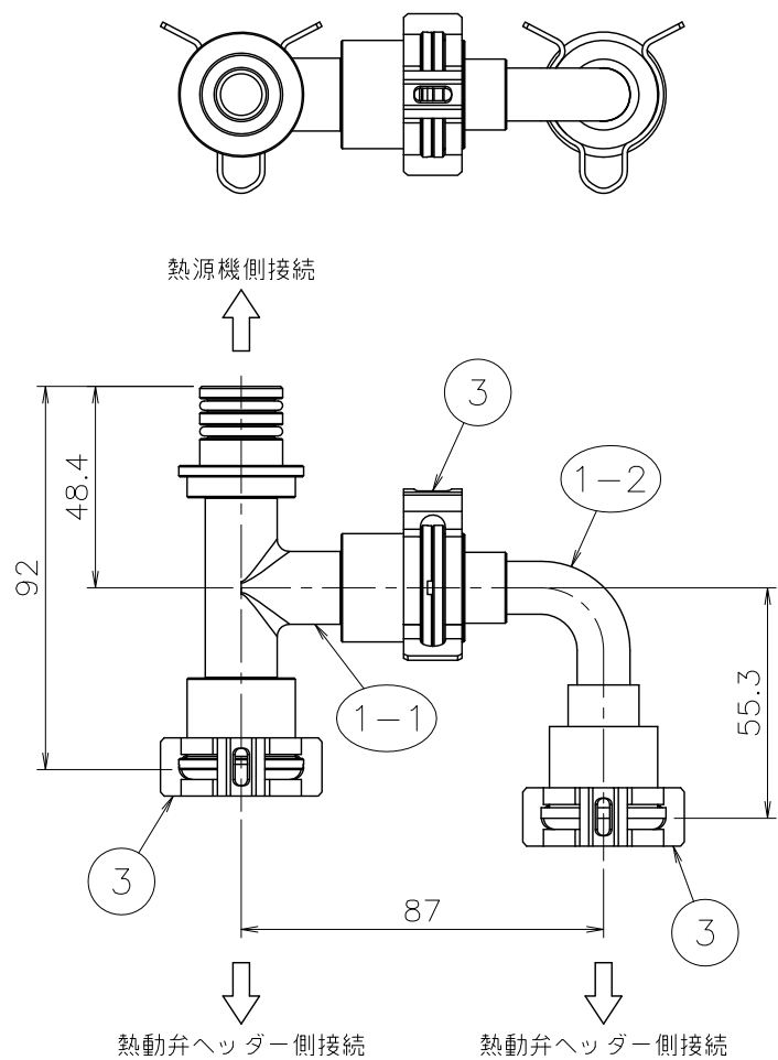
① ヘッダー分岐継手 接続状態図
