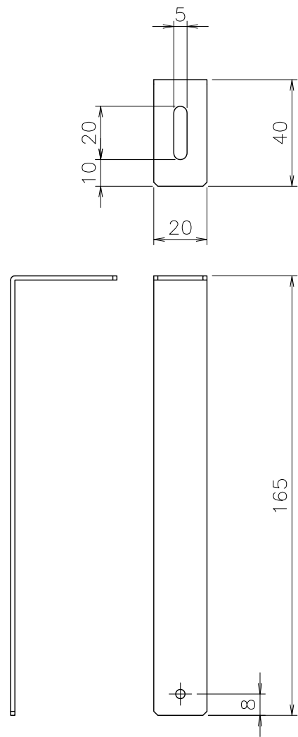
② 熱動弁取付金具
