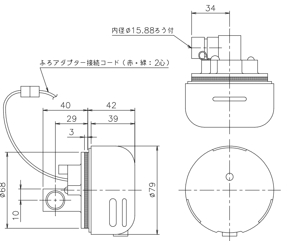
ふろアダプターDX-TL型-L
