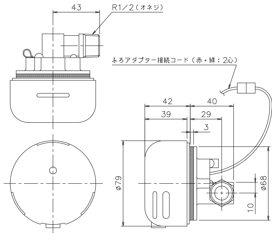
ふろアダプターDX-F型-R
