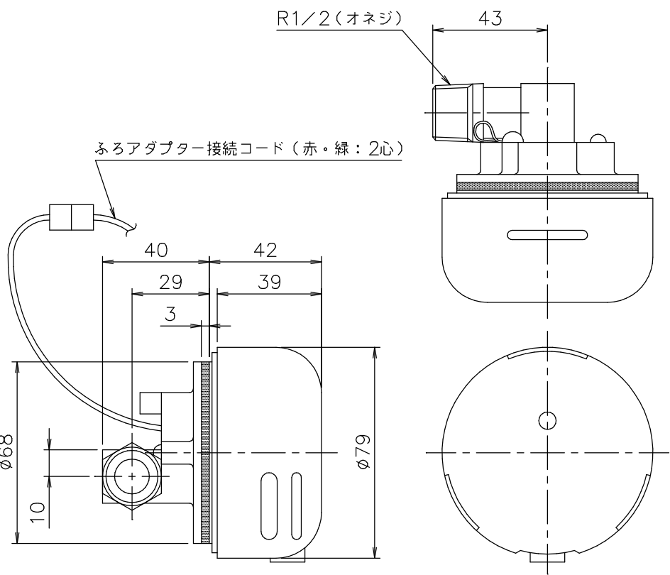
ふろアダプターDX-F型-L
