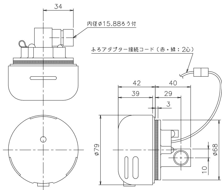
ふろアダプターDX-TL型-R
