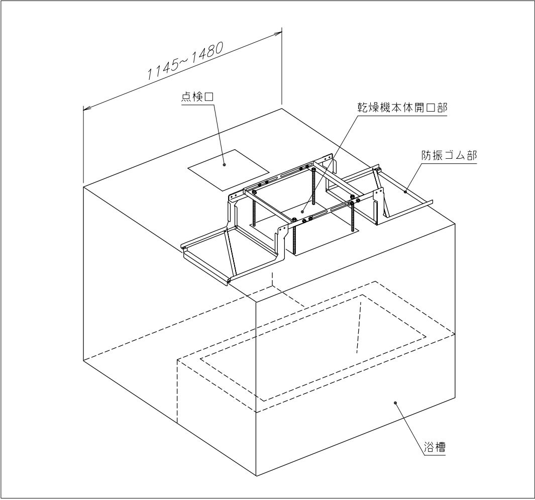
■後付け架台設置参考図
