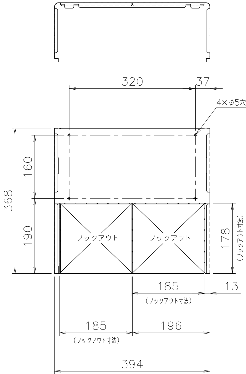
■配管カバーステー（尺度1／6）
