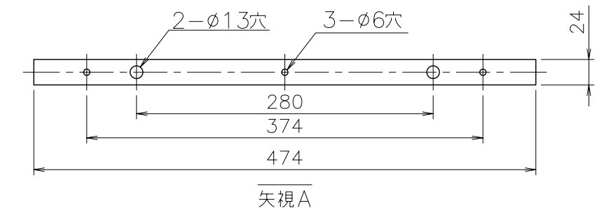
■配管カバー下後板 壁面取付ピッチ
