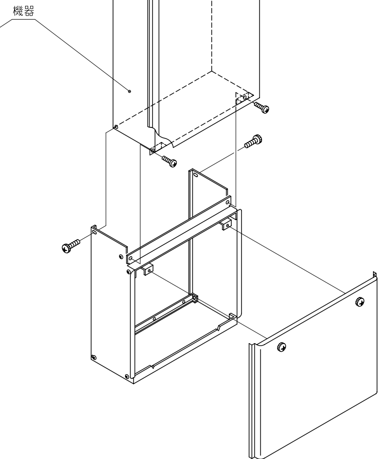
■配管カバー下後板 壁面取付ピッチ
