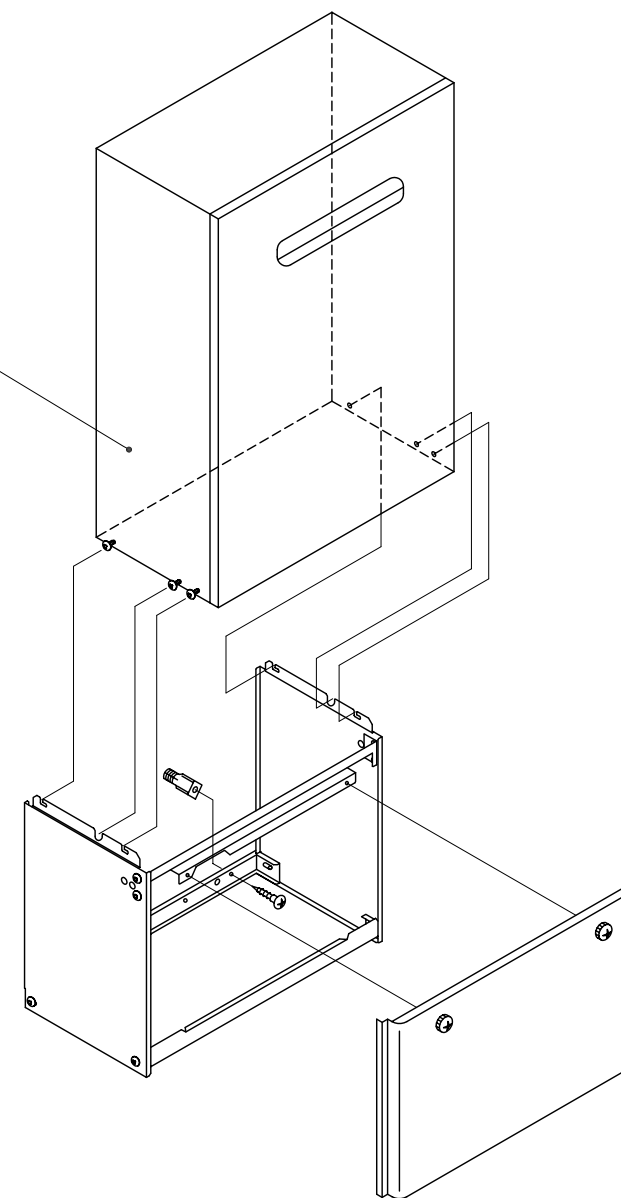
■組立図（概略）
