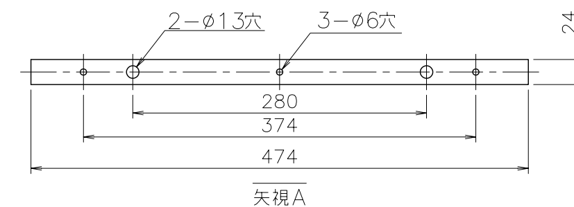
■配管カバー下後板 壁面取付ピッチ
