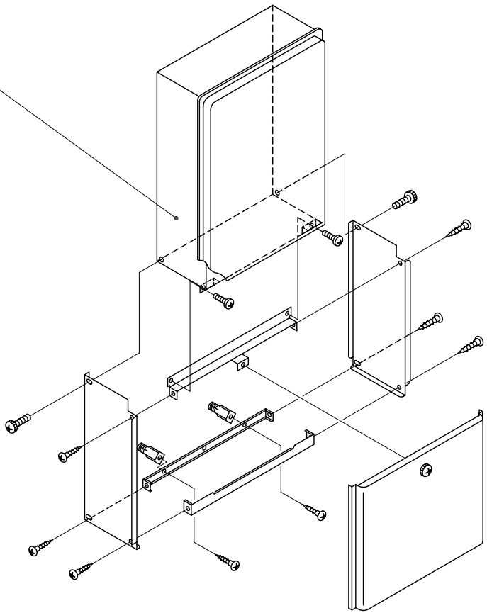
■組立図（概略）
