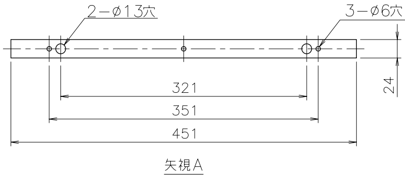
■配管カバー下後板 壁面取付ピッチ
