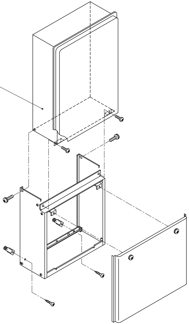
■配管カバー下後板 壁面取付ピッチ
