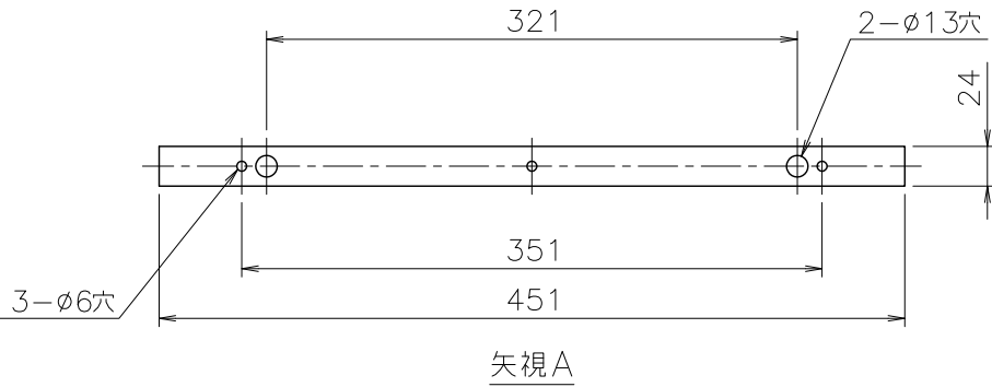
■配管カバー下後板 壁面取付ピッチ
