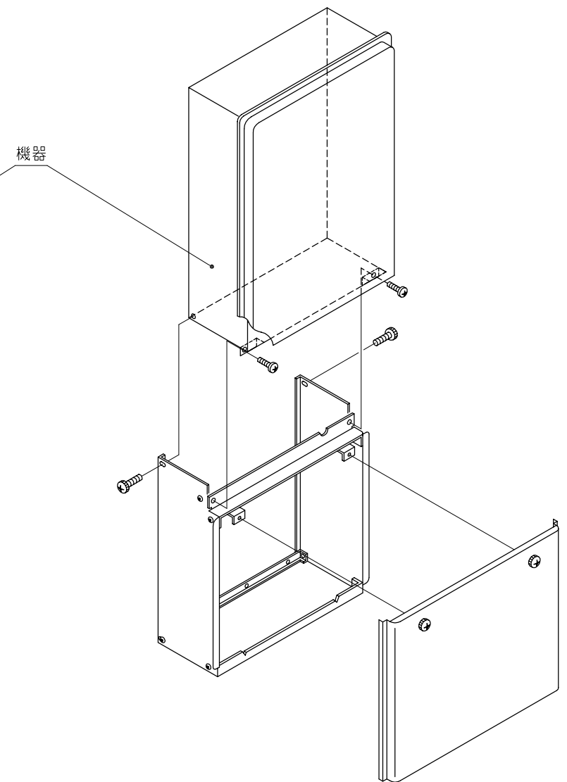
■配管カバー下後板 壁面取付ピッチ
