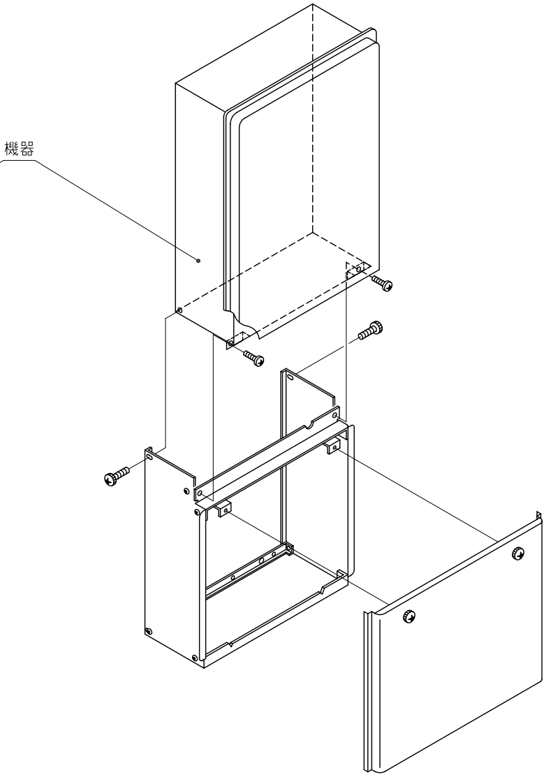
■配管カバー下後板 壁面取付ピッチ
