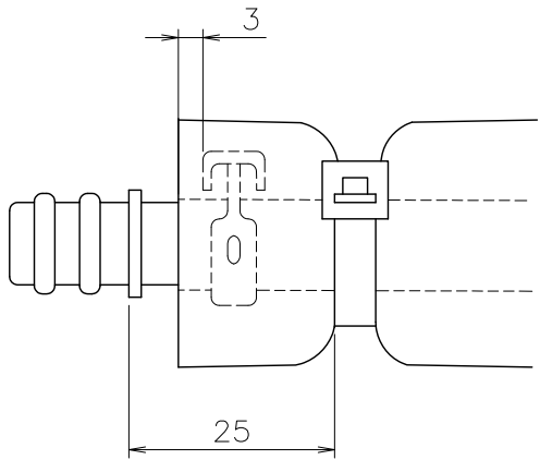
■ PE管ヘッダー継手部 部品組付け位置詳細図（尺度1／1）
