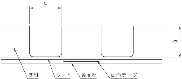
■ A-A断面拡大図（尺度2／1）
