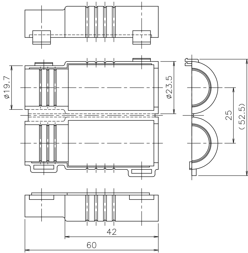
④ ワンタッチカバー φ7用 色：アイボリー 材質：軟質PP
