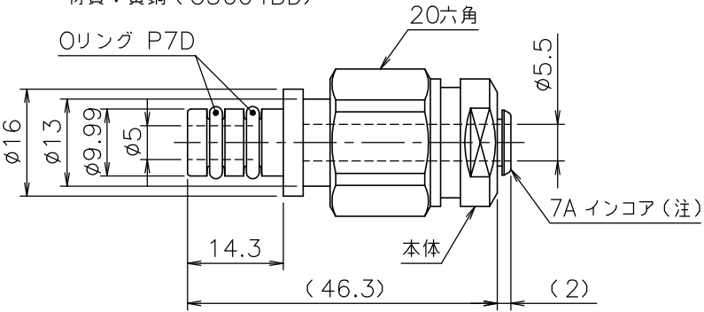
③ CHP1-7W MP 材質：黄銅（C3604BD）
