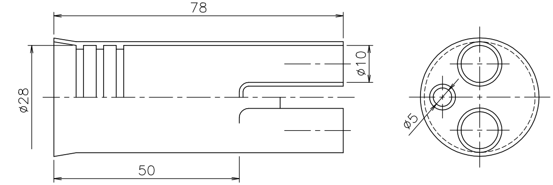
② CHP2-7W MP 材質：黄銅（C3604BD）
