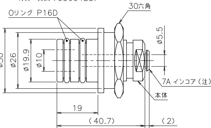
② CHP2-7W MP 材質：黄銅（C3604BD）
