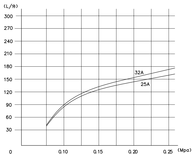
ステンレス吐水口 流量線図
